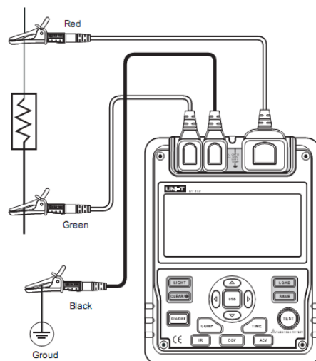
Rysunek 5. Pomiar rezystancji izolacji
