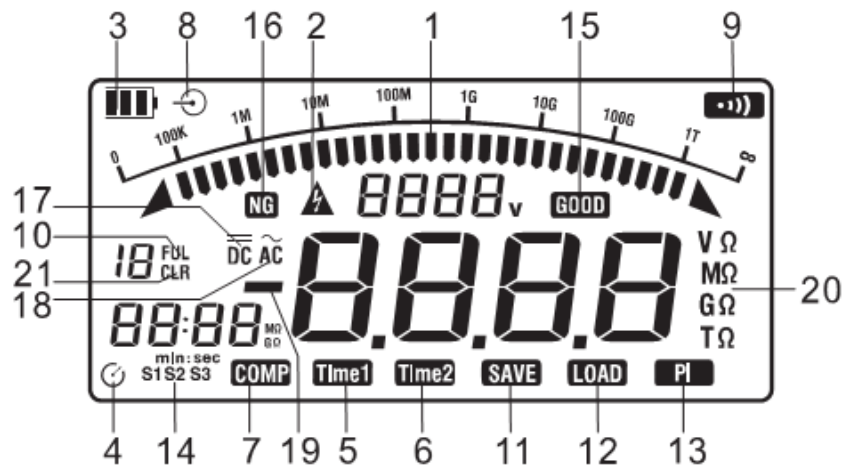
Rysunek 3. Symbole wyświetlacza.
