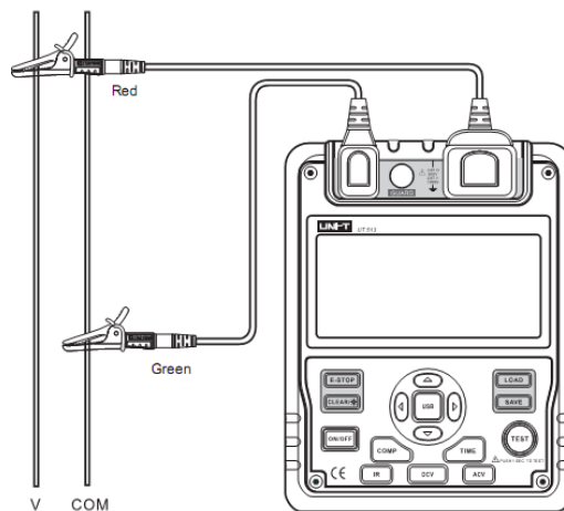
Rysunek 4. Pomiar napięcia
