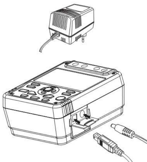
Rysunek 7. Sposób połączenia interfejsu USB
