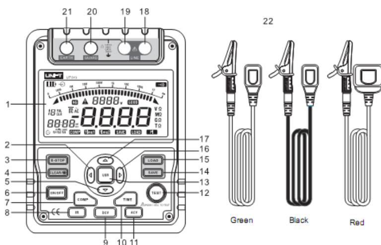
Rysunek 1. Budowa ogólna miernika
